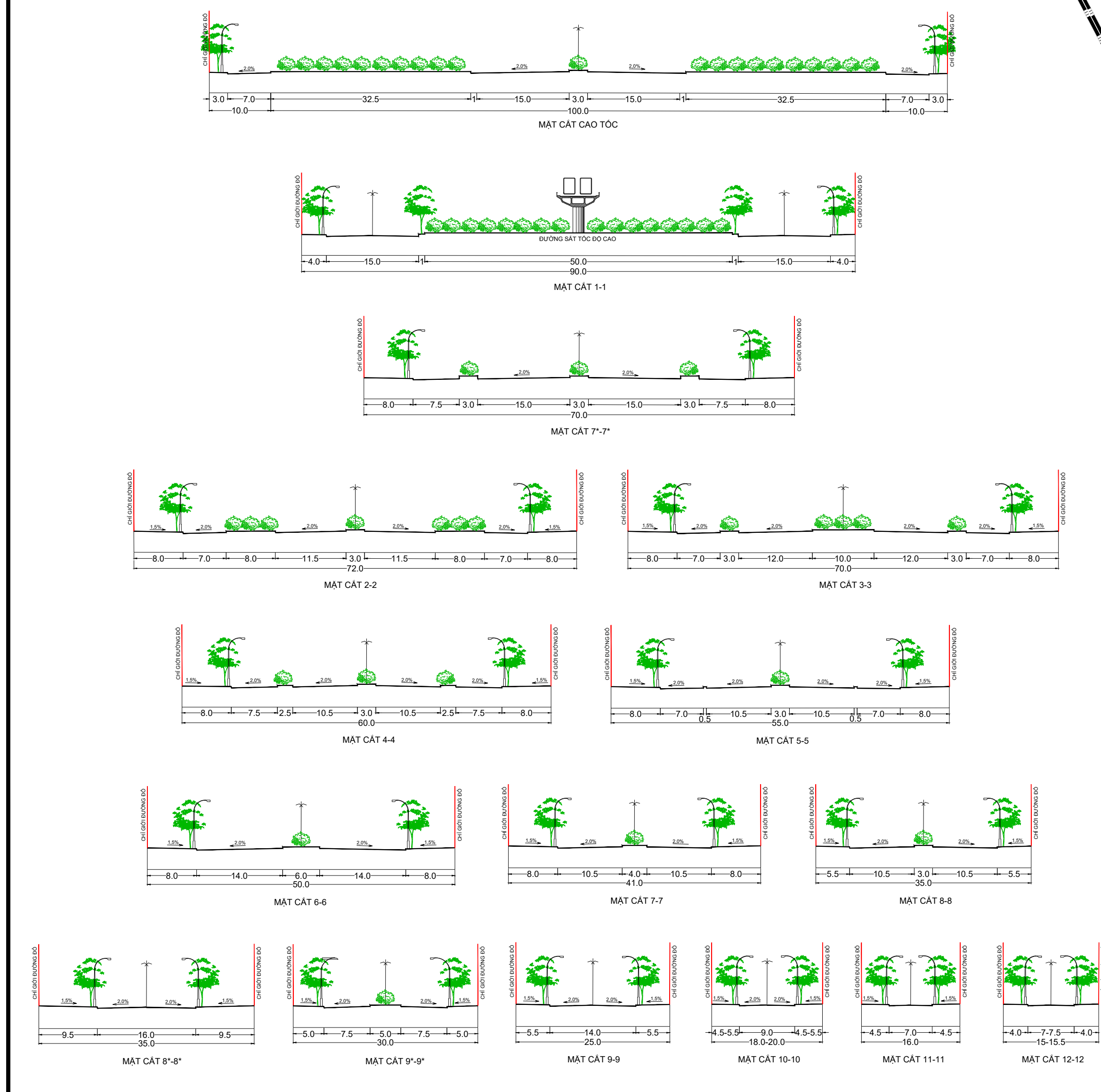
MẶT CÁT NGANG ĐIỂN HÌNH
